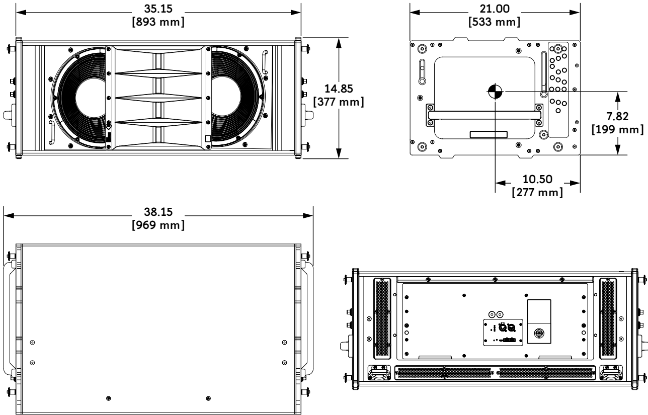
LYON-W Dimensions
