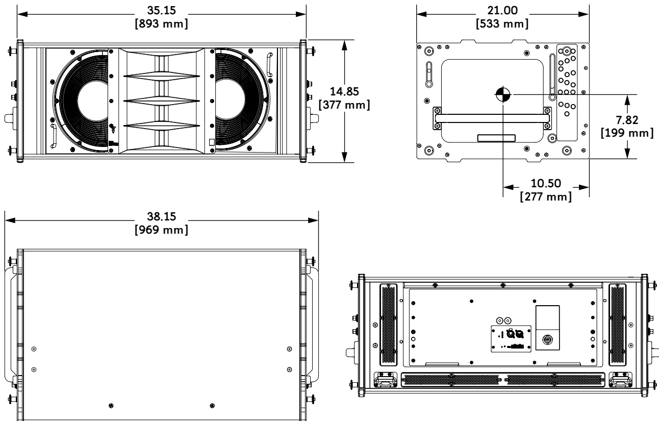
LYON-M Dimensions
