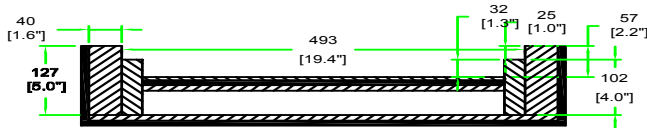
A-A VIEW
